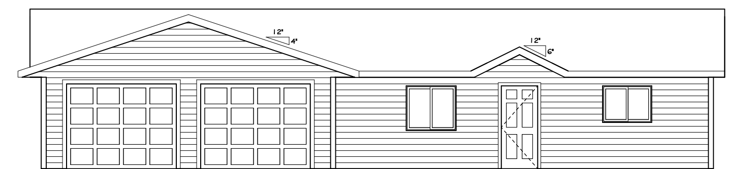
4 FRONT A1 1/4" = 1'-0"
