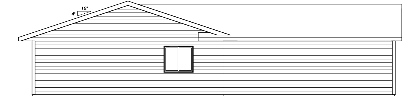
3 LEFT AI 1/4" = 1'-0"
